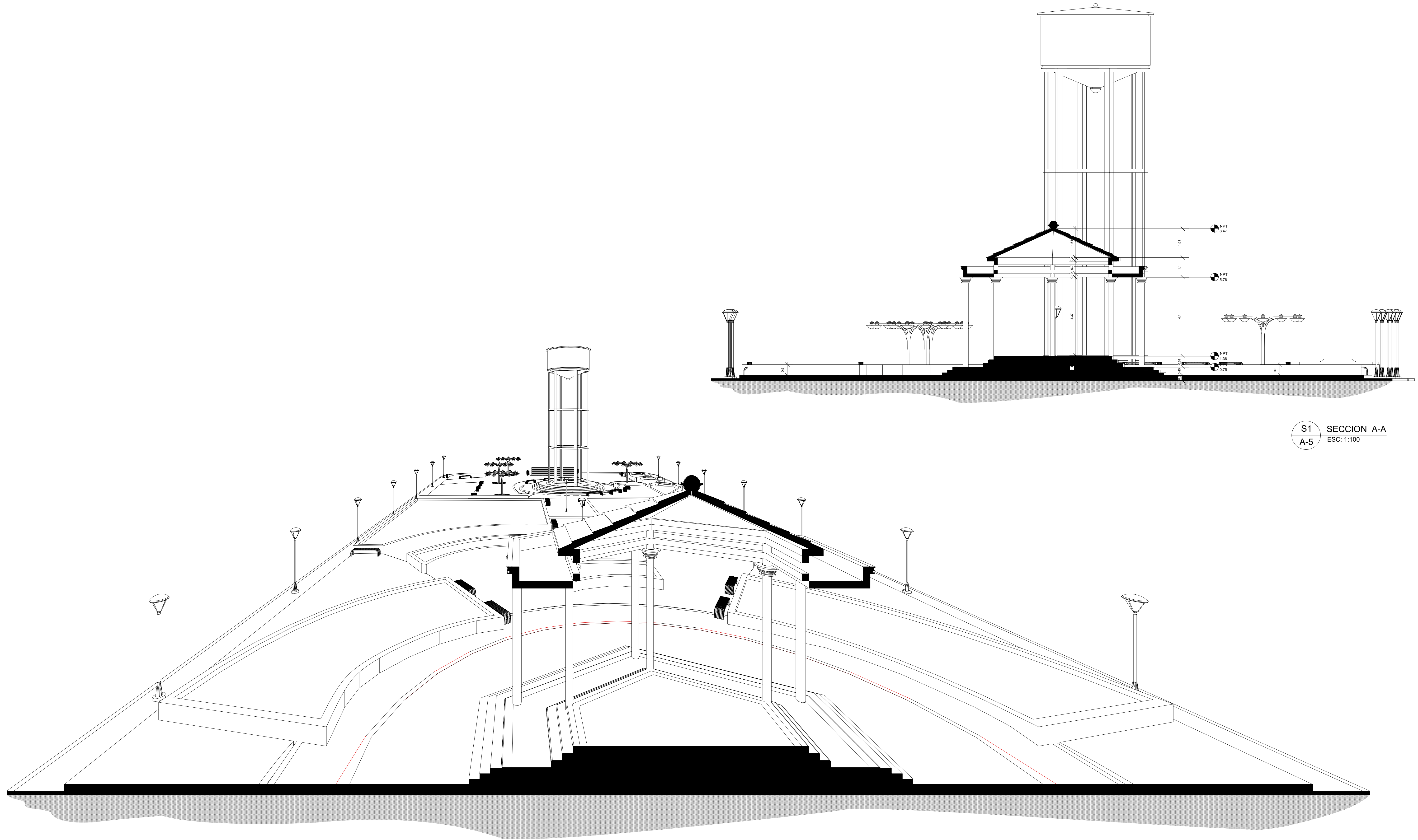
DS1 SECCION A-A ESC: 1:50
